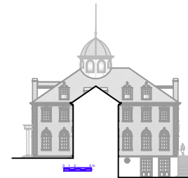
Elevation 04
